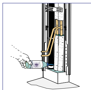
CombiSjakt tett med CombiTett
