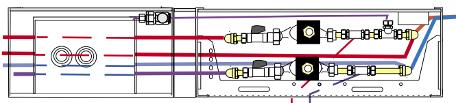
Magnetventiler i S-modul
