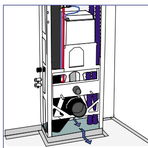
K47 CombiKassett tett med CombiTett
