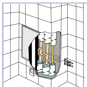
Gipssjakt forseglet med CombiTett i sjaktbunnen samt Indicator lekkasjevarsler
