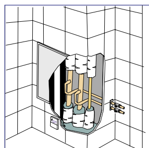
Gipsschakt förseglad med CombiTät i schaktbotten samt Indicator läckagevarnare
