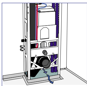
K47 CombiKassett tätad med CombiTät
