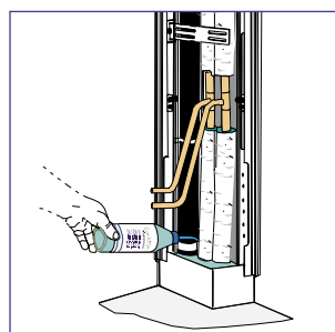
CombiSchakt tätad med CombiTät
