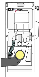
TM-vattenlås WC
