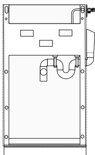
TM-vattenlås TS
