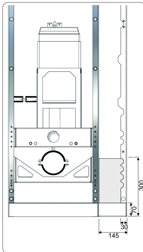
Håltagningszon i front
