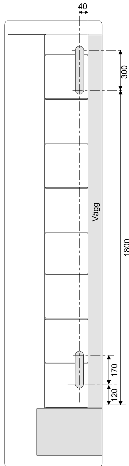
Håltagningszon gavel
